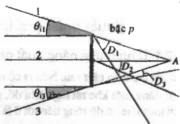
Hình 20. Cách tử không cho một ảnh rõ nét của một vật đơn sắc do A. Các chùm sáng 1, 2, và 3 có những góc tới và những góc lệch khác nhau. Chúng không cắt nhau ở lân cận của cùng một điểm. Do vậy, cách tử không thích hợp để cho ta một ảnh đơn sắc, rõ nét của A.
