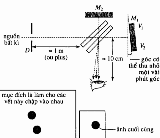
Hình 5. Điều chỉnh hình học sự song song của hai gương nhờ các ốc vít V_1 và V_2 , bằng quan sát trực tiếp bằng mắt thường.
