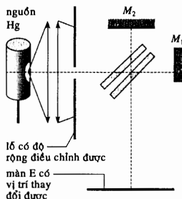
Hình 7. Sơ đồ nghiên cứu sự tương phản của các vân giao thoa.
