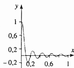
Hình 41b. Đồ thị mô tả sự biến thiên của độ tương phản \Gamma : \operatorname{sinc}(\pi z)
