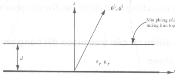
b) Mặt cắt ngang của cấu trúc mạch dải hình dạng bất kỳ có mặt phẳng kim loại ở đế
