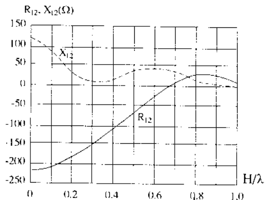
Hình 6.20. Trở kháng tương hỗ của chấn tử và anten khung tròn:
