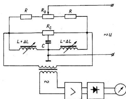
Hình 2.15 Mạch đo cảm biến điện cảm
