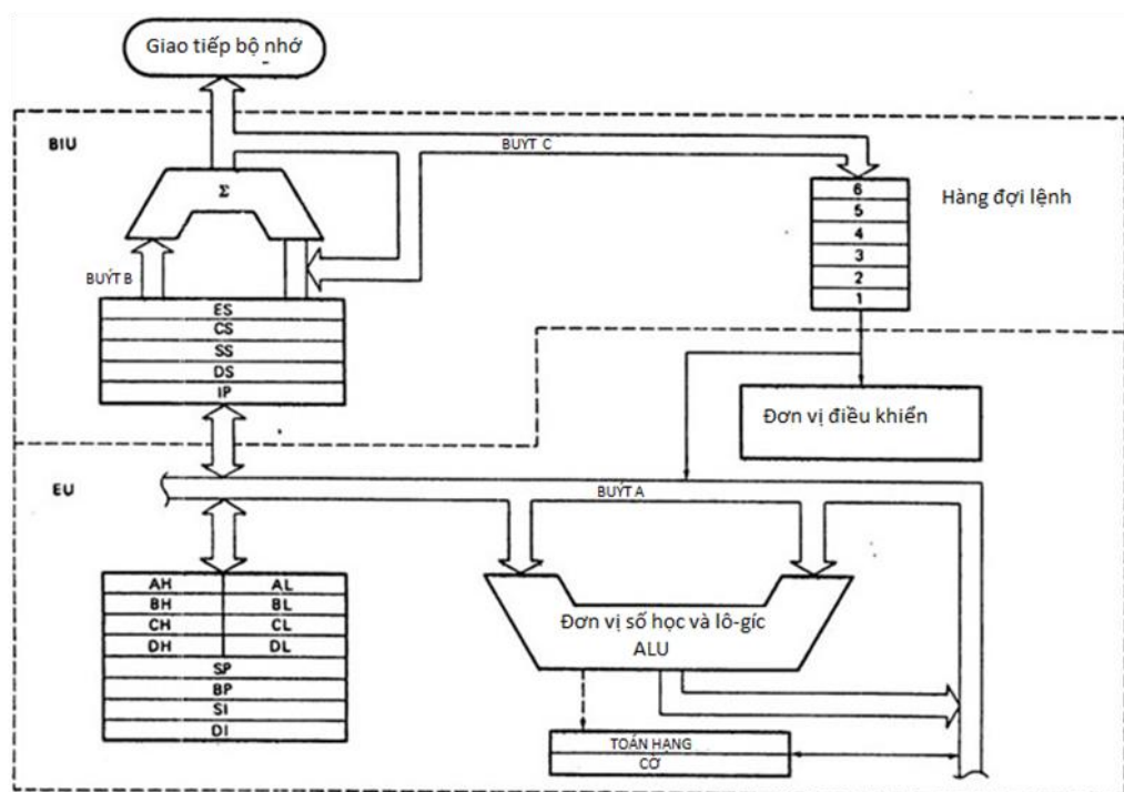
Hình II-1. Sơ đồ khối 8086
