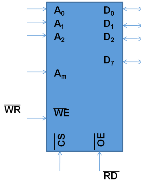
Hình IV-8. Vi mạch nhớ khái quát
