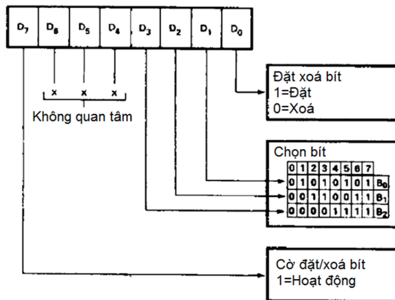
Hình IV-26. Đặt xoá các tín hiệu điều khiển trên cổng C
