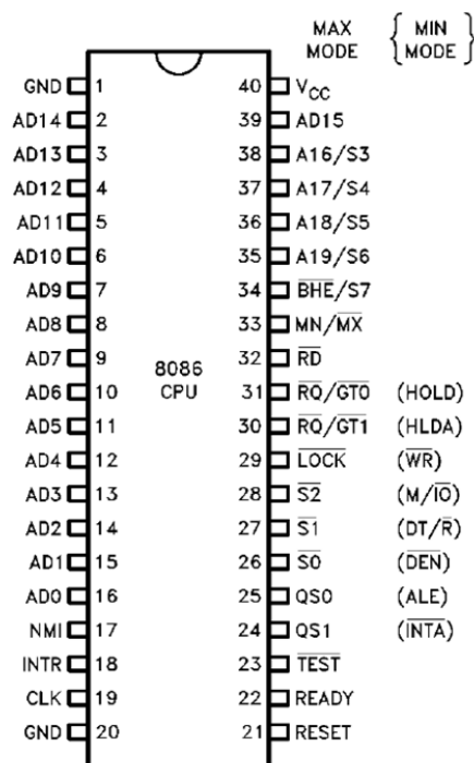
Hình IV-1. Tín hiệu 8086
