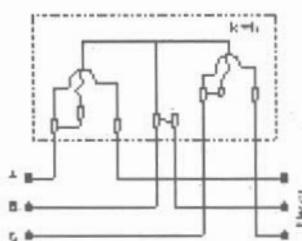
Hình 4.16. Sơ đồ nối dây đồng hồ đo điện năng 3 pha 2 phần tử
