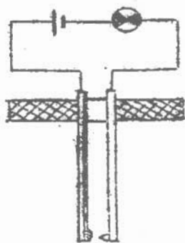
Hình 5.1: Nhiệt kế cơ khí dùng làm rơ le khống chế nhiệt độ hoặc cho tín hiệu nhiệt độ
