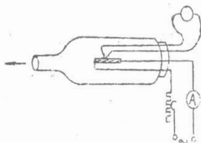
Hình 5.13: Chân không kế nhiệt điện trở
