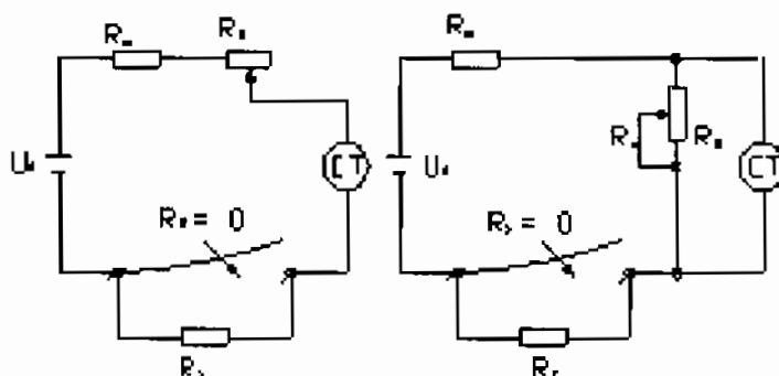
Hình 4.21. Sơ đồ ômmét chỉ thị mắc nối tiếp
