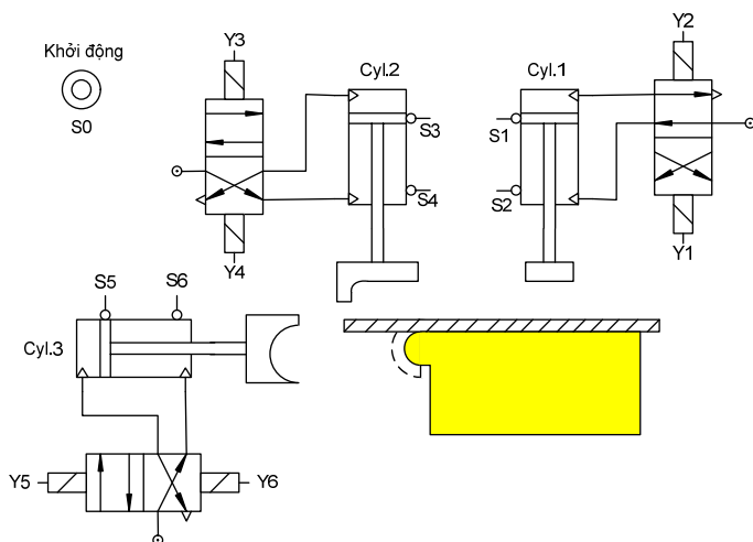
Hình 11.15: Sơ đồ công nghệ máy uốn thanh kim loại
