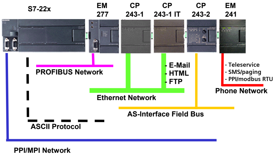
Hình 4.4: Khả năng truyền thông của PLC S7-200
