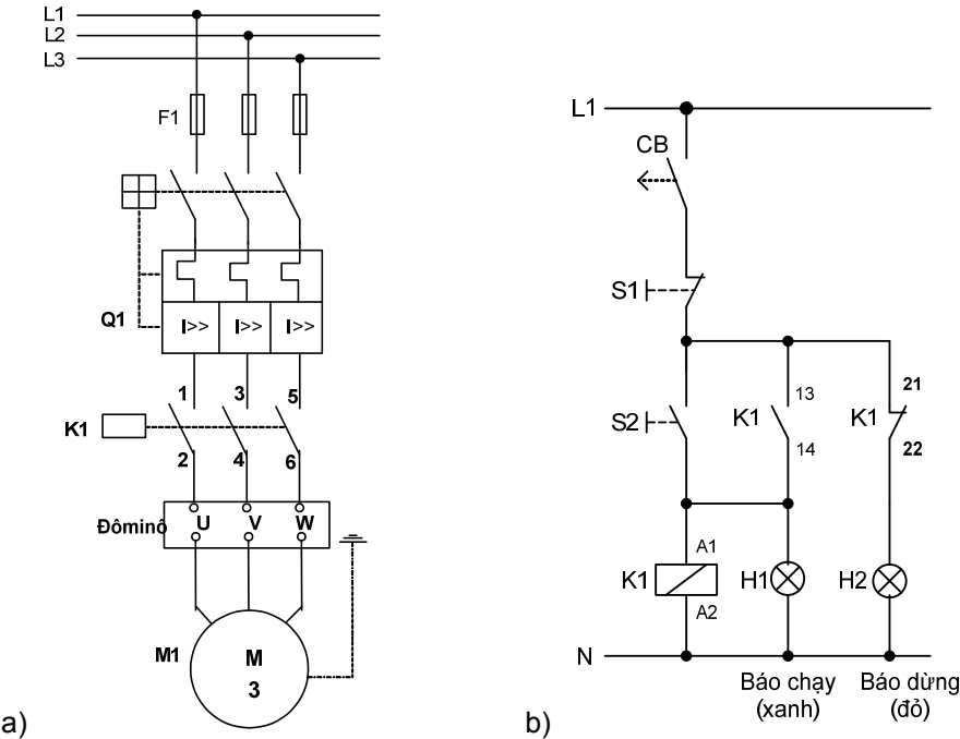
Hình 7.14 Mạch ON/OFF động cơ dùng contactor.
