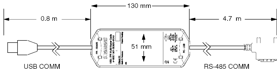
Hình 5.4: Hình dáng cáp USB/PPI.
