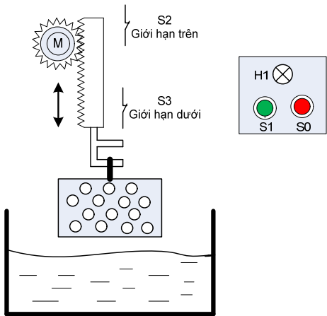
Hình 10.3 Sơ đồ công nghệ bể ăn mòn
