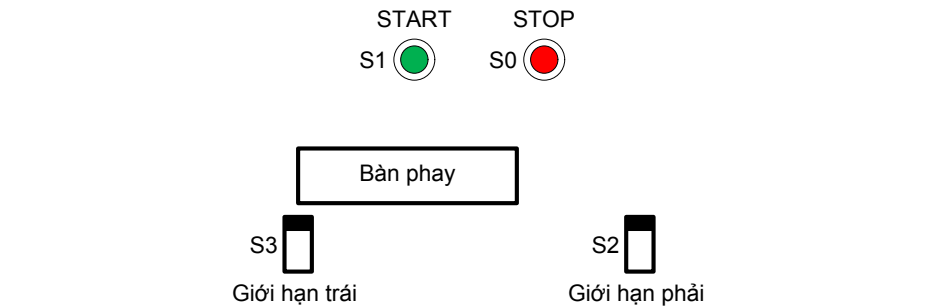
Hình 11.8: Sơ đồ công nghệ máy phay đơn giản
