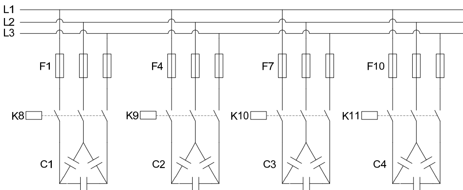
Hình 13.1: Mạch động lực của thiết bị đóng tự bù.
