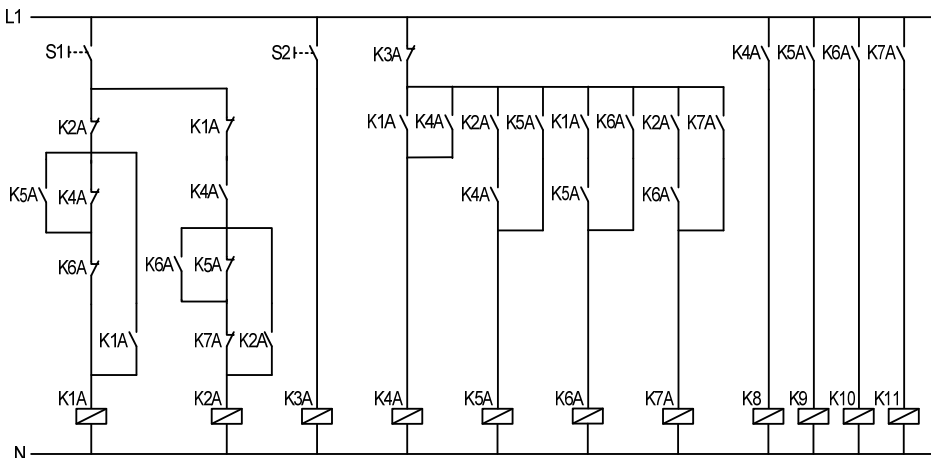
Hình 13.2: Sơ đồ mạch điều khiển bằng contactor thiết bị đóng tự bù
