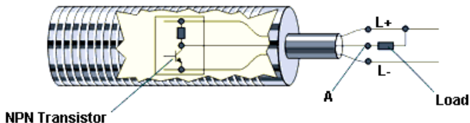
Hình 3.3: Cảm biến NPN (cảm biến “rút dòng”).
