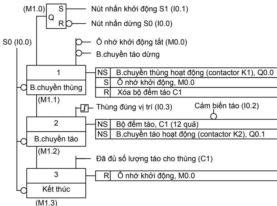
Hình 11.11: Sơ đồ điều khiển theo trình tự bằng chuyển đếm tải
