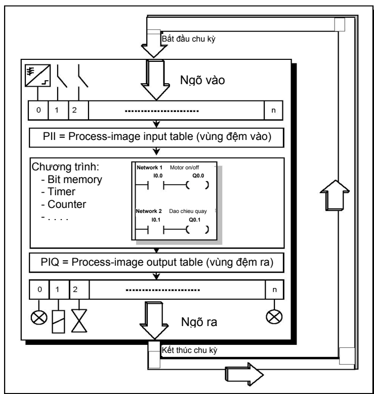
Hình 2.8: Chu kỳ quét trong PLC
