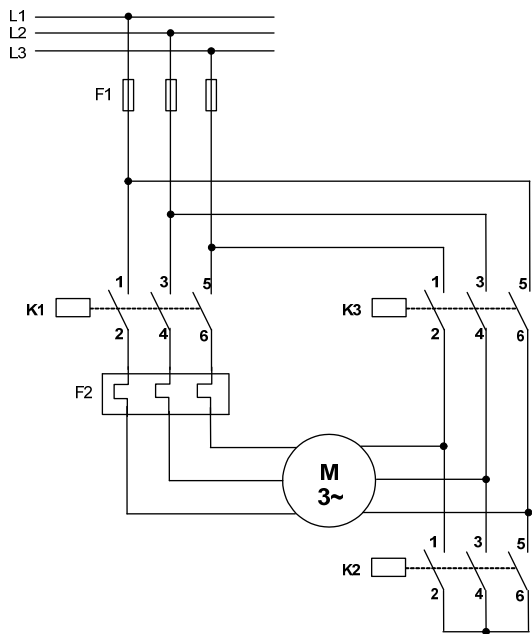
Hình 9.8: Mạch động lực khởi động sao-tam giác.
