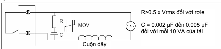
Hình 12.19: Mạch bảo vệ ngõ ra relay có nguồn điều khiển AC.
