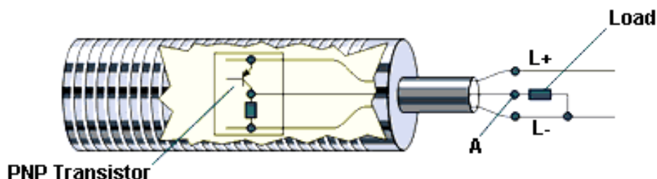
Hình 3.4: Cảm biến PNP (cảm biến “sourcing”)
