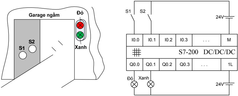
Hình 10.2: Sơ đồ Ragare ngầm và sơ đồ nối dây PLC
