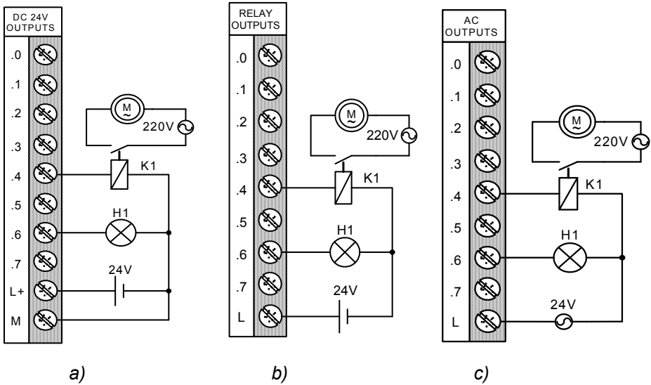
Hình 5.9: Kết nối dây ngõ ra PLC với cơ cấu chấp hành
