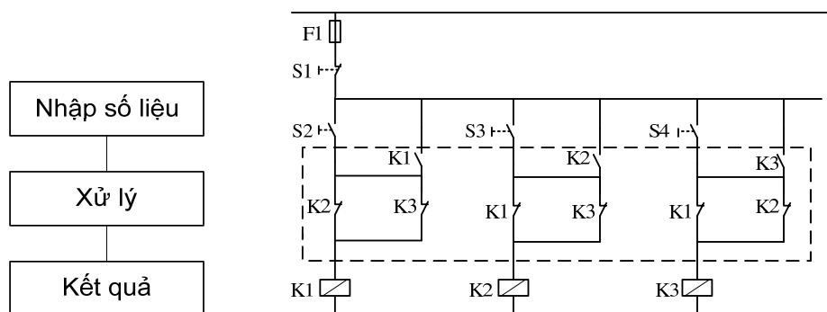
Hình 2.4: Sơ đồ mạch điều khiển 3 động cơ đã được thay đổi
