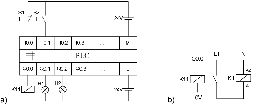
Hình 7.15: a) Sơ đồ nối dây PLC b) Nối relay trung gian với contactor
