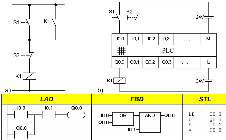
Hình 7.13 Mạch ưu tiên dừng máy:
