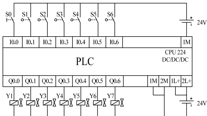
Hình 13.12: Sơ đồ nối dây ngoại vi với ngõ vào ra của PLC
