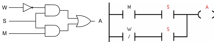
Hình 8.16: Biểu thức Bool và được thực hiện với LAD
